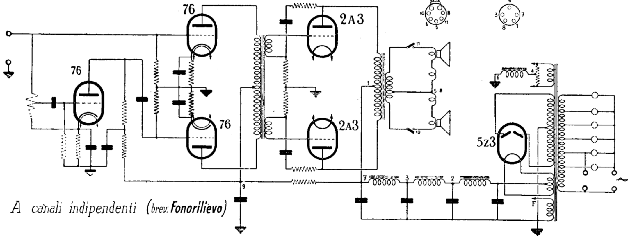
65. — IMCARADIO. — Mod. « Multigamma IF 164 ». — Complesso B. F. 2A3.
